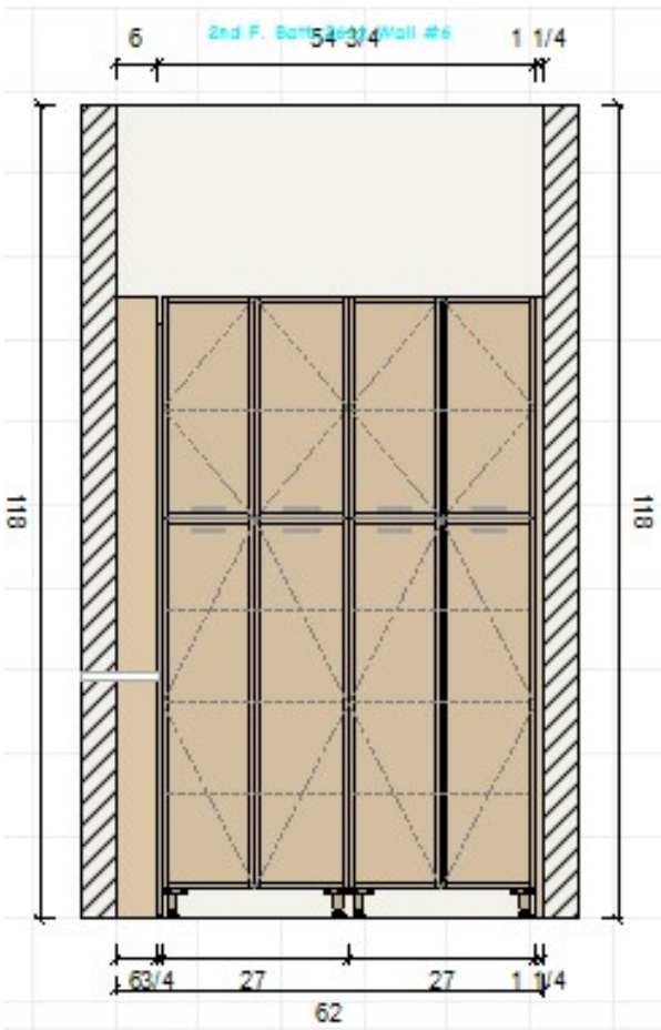
Linen Cab. Elevation
